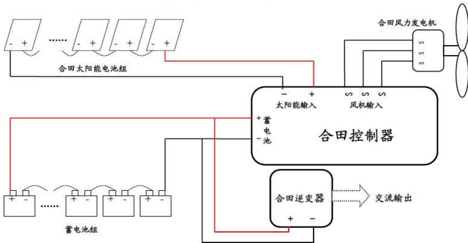
合田新能源风光互补系统连接图
