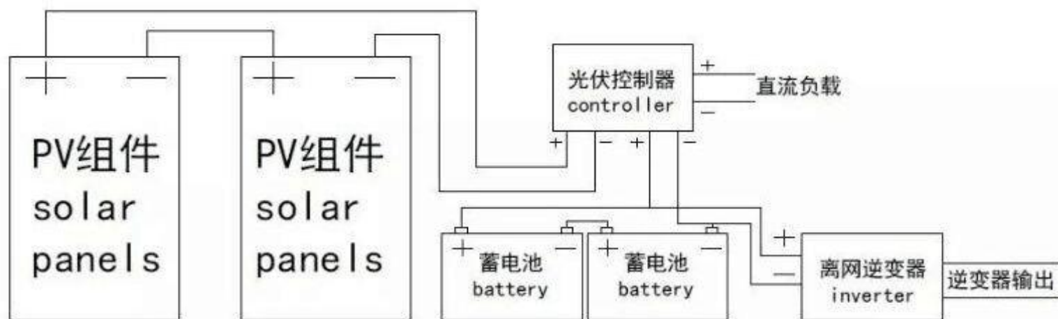
光伏离网交流发电系统裸接拓补图 绍兴合田新能源有限公司
