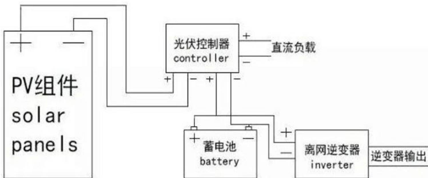
光伏离网交流发电系统裸接拓补图
